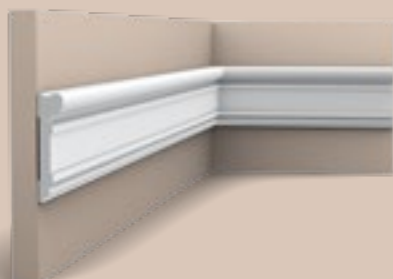
DX119-2300 230 x 9,2 x 2,2 cm Duropolymer®
